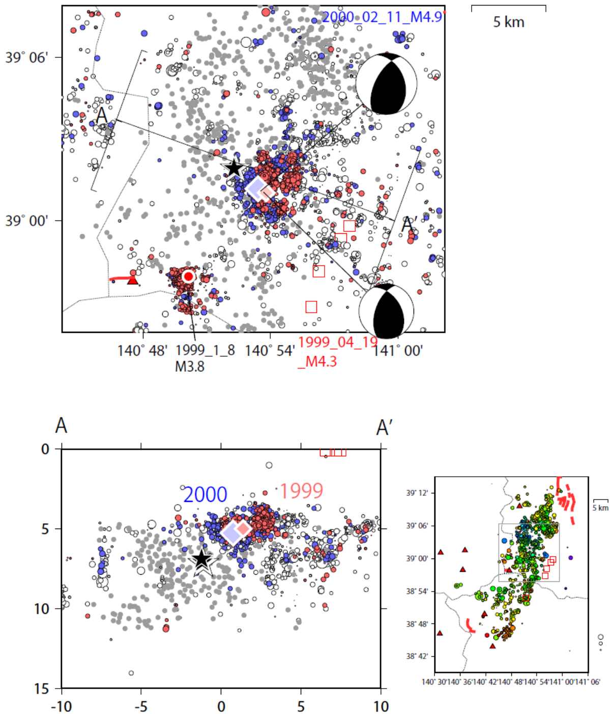
図9. 2008年岩手・宮城内陸地震震源付近における微小地震活動. 岡田・他(2008)による1997年から2008年までの震源分布を示す. 白☆, 黒★, 灰色○は本震, 前震(8:01,8:11), 余震(6/14-17, 20)を示す. 赤は1999年の活動, 青は2000年の活動を示す. 赤◇は, 1999/4/19M4.3の地震, 青◇は2000/2/11 M4.9の地震を示す. 赤線四角は地表地震断層の位置. (上図)震央分布図. 1999/4/19M4.3の地震, 2000/2/11 M4.9の地震のメカニズム解をあわせて示す. (下図)A-A'断面図. 1999年・2000年の地震の余震分布は西傾斜の傾向にあり, 2008年岩手・宮城内陸地震の余震の並びの浅部延長に位置することから, 同一断層面上での活動であると推定される. なお, 1999年・2000年の震源域(余震域)では, 今回の地震の余震活動は低調である.
