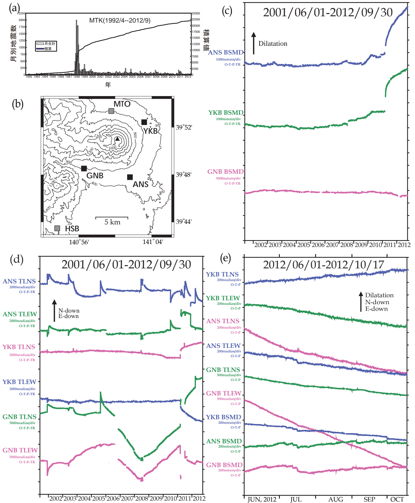
図1. 岩手山周辺における歪・傾斜変動連続記録。(a) 月別地震数の変化(1992年4月~2012年9月), (b) 観測点配置, (c) 2001年6月~2012年9月における歪変動, (d) 傾斜変動, (e) 2012年6月1日~2012年10月17日の歪・傾斜変動. BSMD: 体積歪, TLNS: 傾斜南北成分, TLEW: 傾斜東西成分. (c), (d)は潮汐・気圧・トレンド補正済. (e)は潮汐・気圧のみ補正済. トビをともなう変動は大きな地震の影響あるいは降水の影響. 2011年3月以降は3月11日M9.0と余震などの影響が大きいために不明確ではあるが, 有意な火山性的変動はないと考えられる. 地形図の作成には国土地理院発行の数値地図を使用した.
