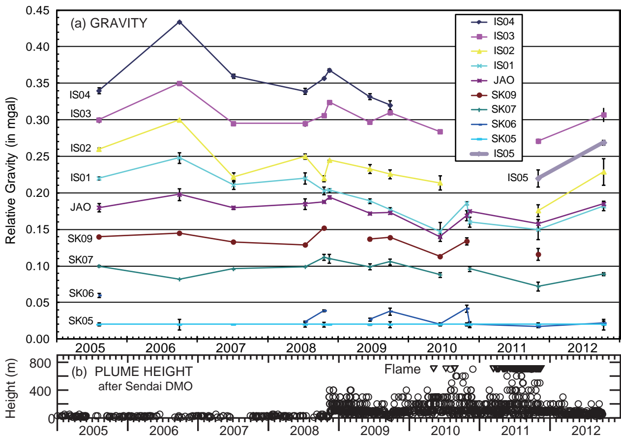
図2. (a) 基準点 SK05 に対する相対重力値の時間変化と (b) 噴気活動(2005年～2012年)。
