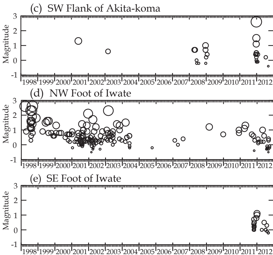
図2. 岩手火山・秋田駒ヶ岳火山地域における、2011年東北地方太平洋沖地震(M9.0)前後の地震活動の比較。(a)地震後1年半(2011年3月~2012年9月), ならびに, (b)地震前約2年間(2009年1月~2011年2月)の震源分布. 緑の円c~eはM9.0地震以後に地震活動が活発化した地域. (c)~(e)上記の活動域における地震活動のM-T図(1998年1月~2012年9月). (c), (d)では2011年2月以前にも地震活動が認められるが, (e)の活動は2011年後半に生じたものである. 今後の推移に注目したい.
