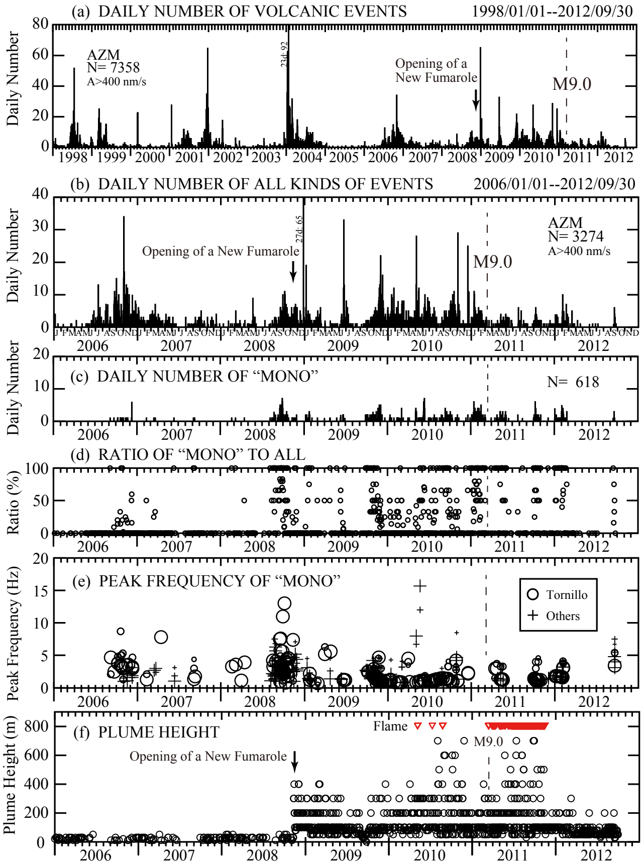
図1. 吾妻火山地域における地震活動(a)～(e)と噴気活動(f). (a)1998年1月～2012年9月, (b)2006年1月1日～2012年9月30日の地震活動の推移. (c)その中の「単色」地震の活動, (d)全地震数に対する「単色地震」数の割合, (e)「単色地震」の卓越周波数の時間変化, (f)日別最高噴気高の時間変化(仙台管区気象台による). 逆三角形は硫黄自然発火を示す. 2010年までは「単色地震」の活動と噴気活動が関連. 噴気活発化の前に多様な卓越周波数の地震が発生. M9.0地震によりこの関係が変化した可能性あり. 2012年3月以降は両活動ともに低下.
