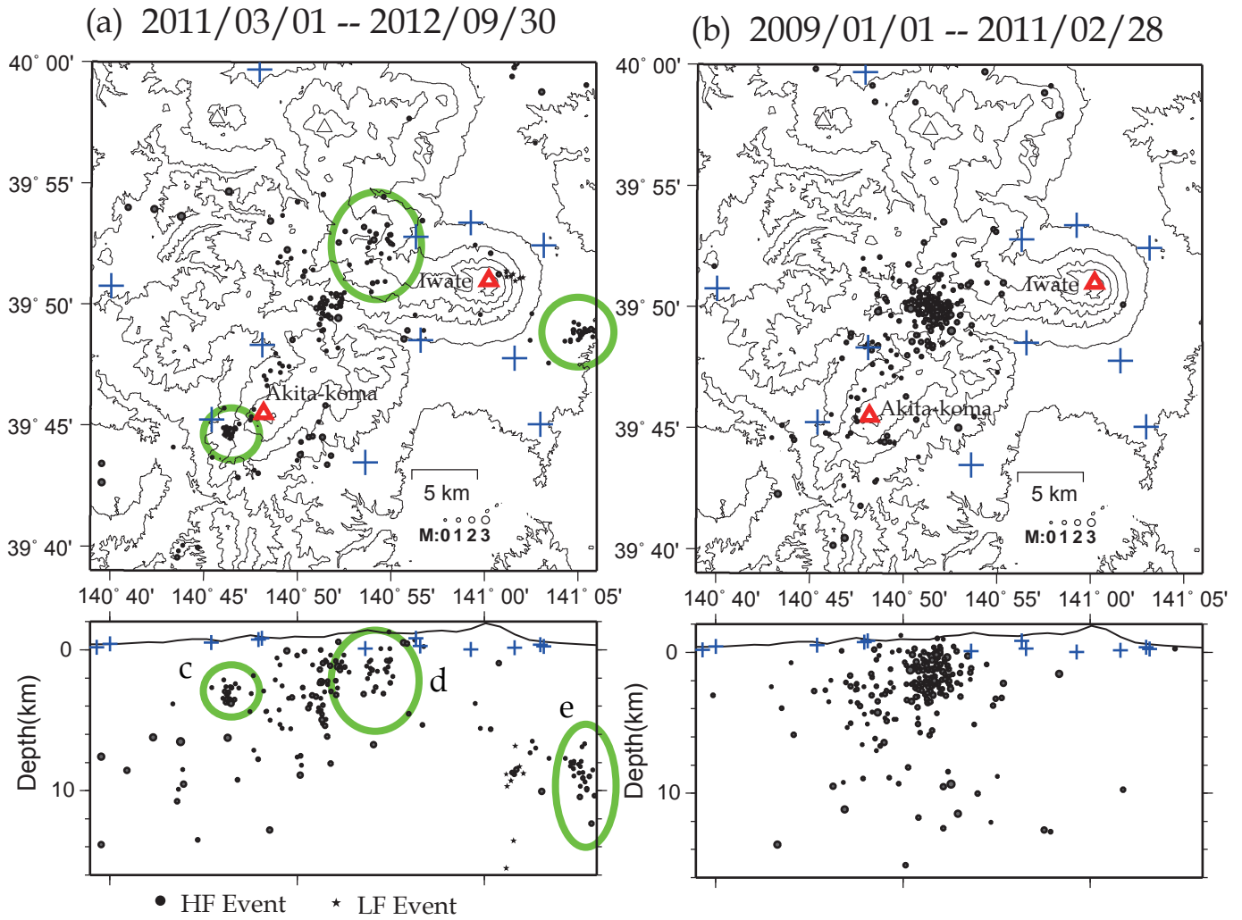
図2. 岩手火山・秋田駒ヶ岳火山地域における、2011年東北地方太平洋沖地震(M9.0)前後の地震活動の比較。(a)地震後1年半(2011年3月~2012年9月), ならびに, (b)地震前約2年間(2009年1月~2011年2月)の震源分布. 緑の円c~eはM9.0地震以後に地震活動が活発化した地域. (c)~(e)上記の活動域における地震活動のM-T図(1998年1月~2012年9月). (c), (d)では2011年2月以前にも地震活動が認められるが, (e)の活動は2011年後半に生じたものである. 今後の推移に注目したい.
