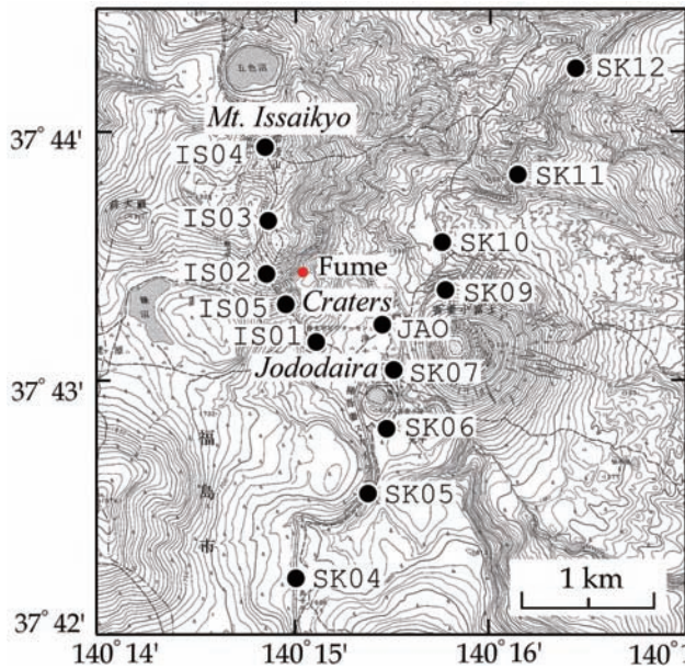
図1. 吾妻火山重力観測網 (地形図は国土地理院発行 1/25,000 地形図を使用)。
